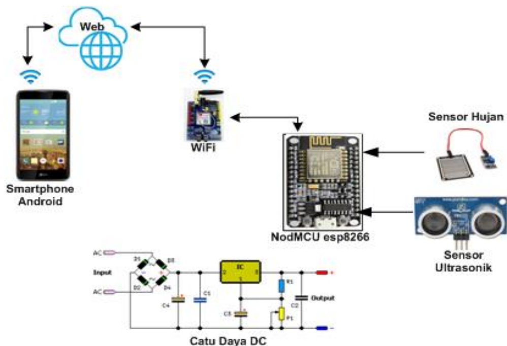
Gambar 1. Blok Diagram Sistem.
